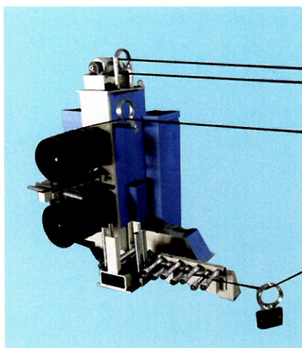
张力架 Tension frame
